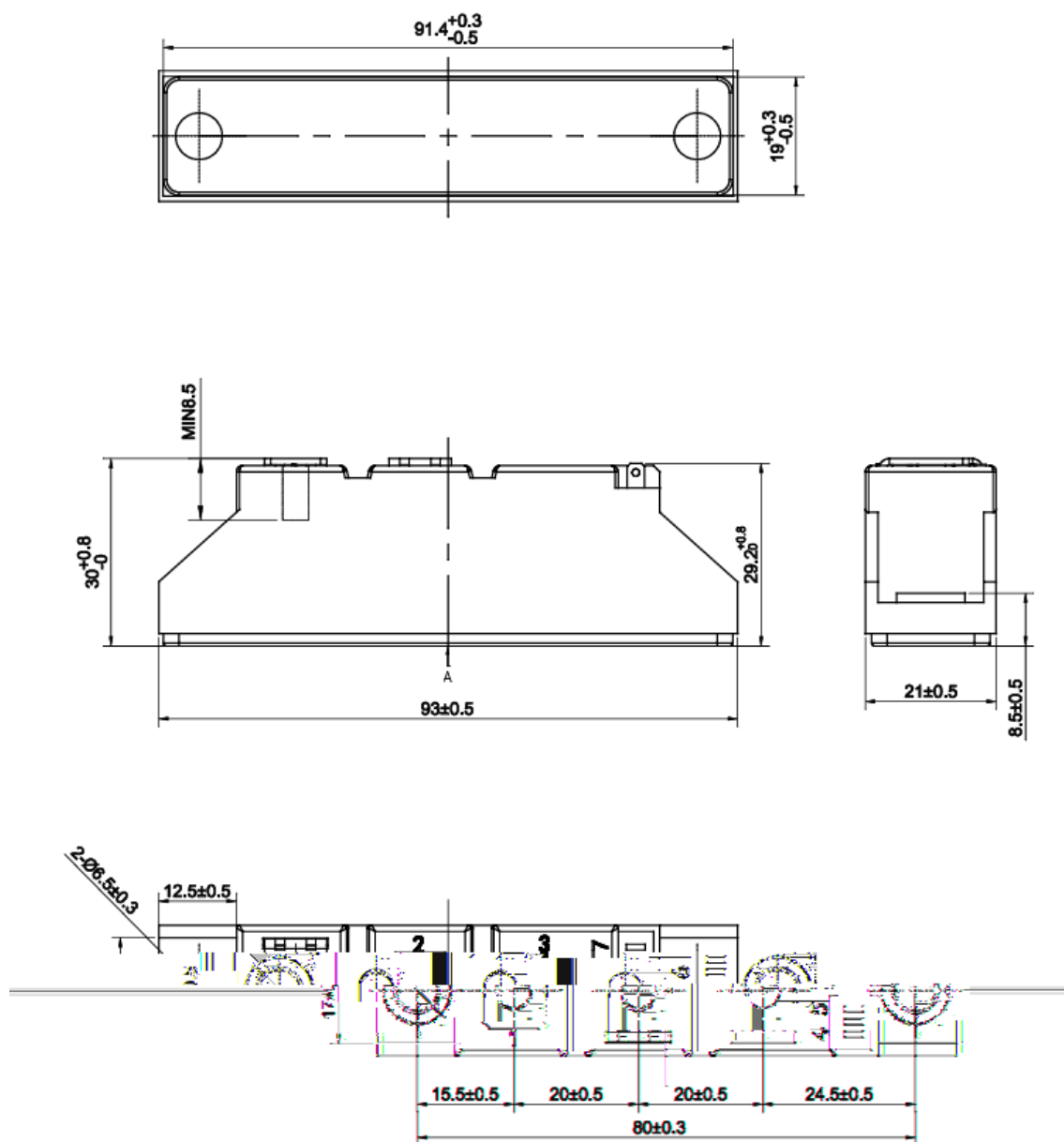
A视图
